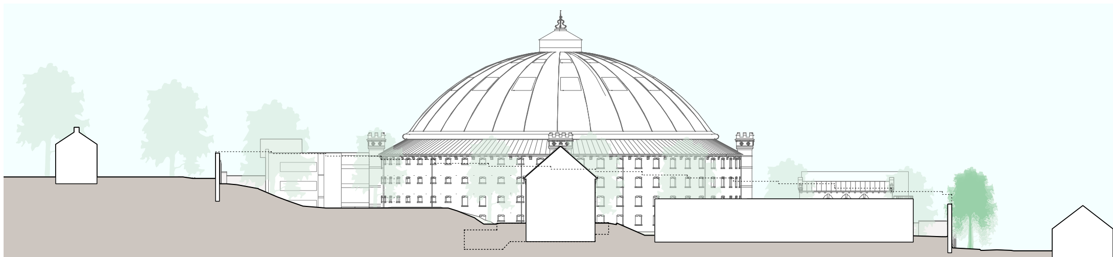
dwarsprofiel in de huidige situatie van het koepelcomplex over het dienstengebouw
